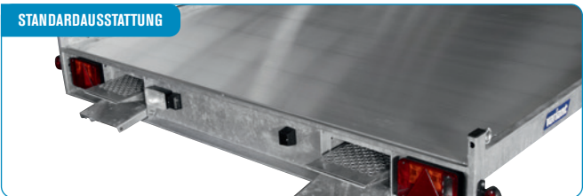
Aluminiumprofilboden in kräftiger Ausführung. Rutschfest und stark. Auffahrampen zur Aufbewahrung im Bohlenschacht unter der Ladefläche. 2,5 Mtr. - 4.000 kg
